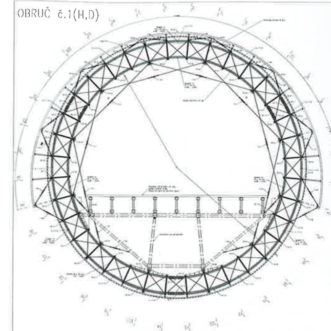
▲ Typický příčný řez vzducholodí (obruč č. 1)
