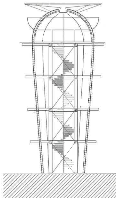
Řez Section
