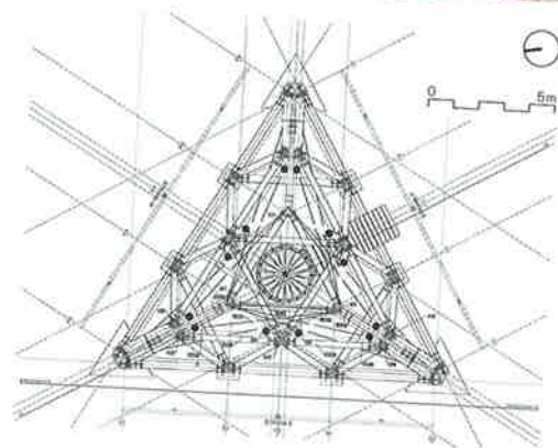
Půdorys
