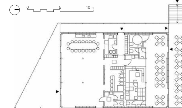
Půdorys 1. NP
