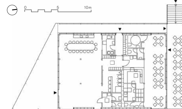
Půdorys 1. NP
