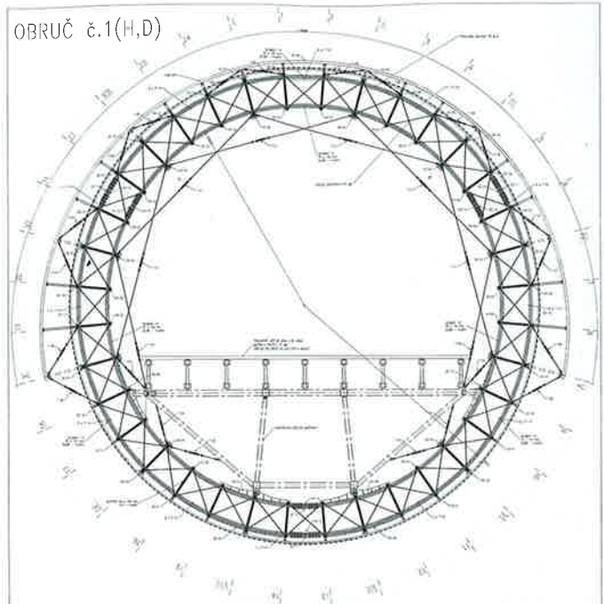
▲ Typický příčný řez vzducholodi (obruč č. 1)
