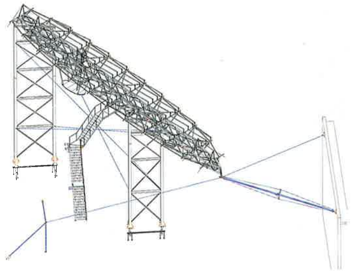
▲ 3D model ocelové konstrukce, na kterou je ukotvena dřevěná konstrukce vzducholodi
